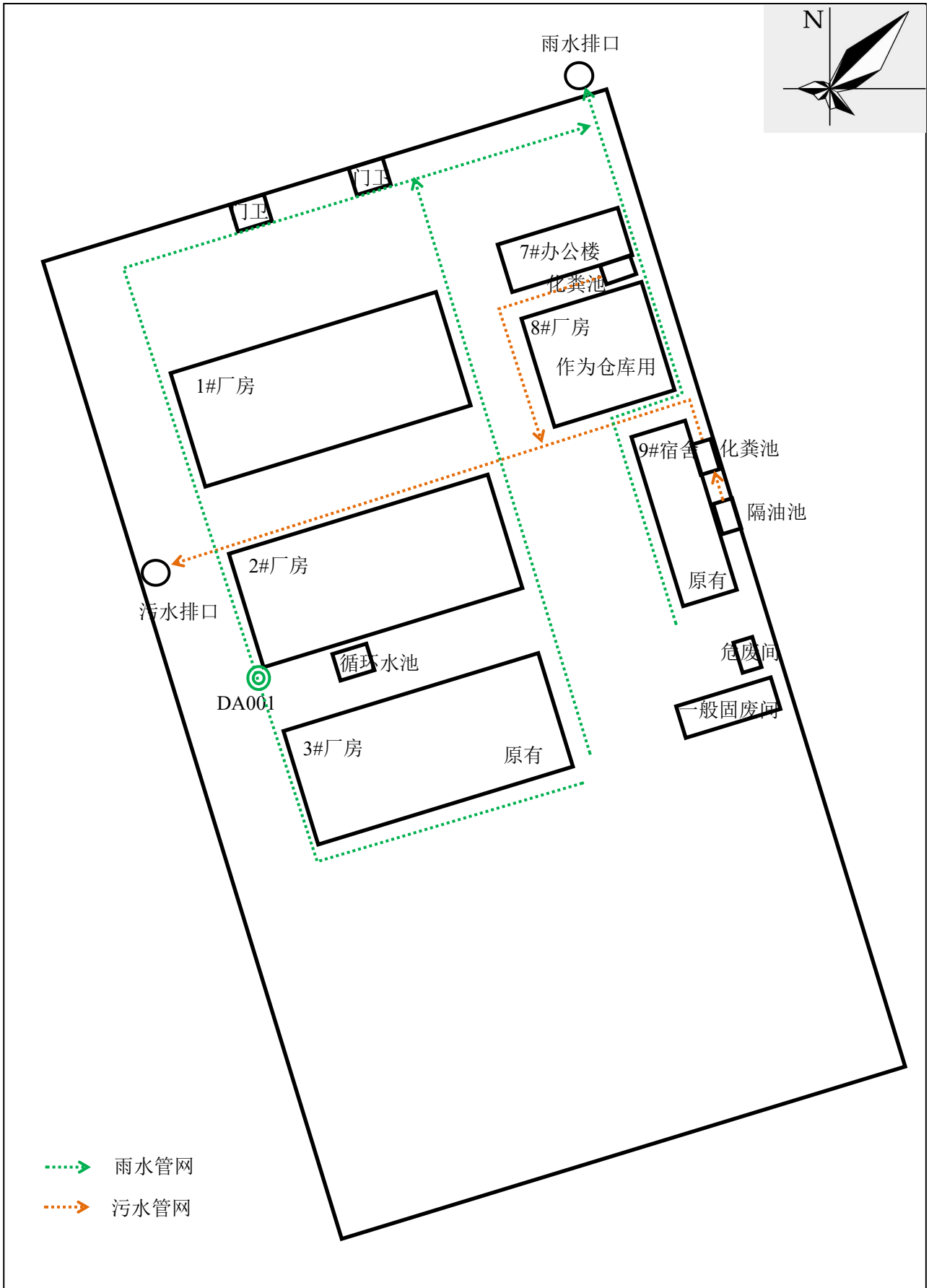
附图3 厂区总平面布置图及雨污管网图
